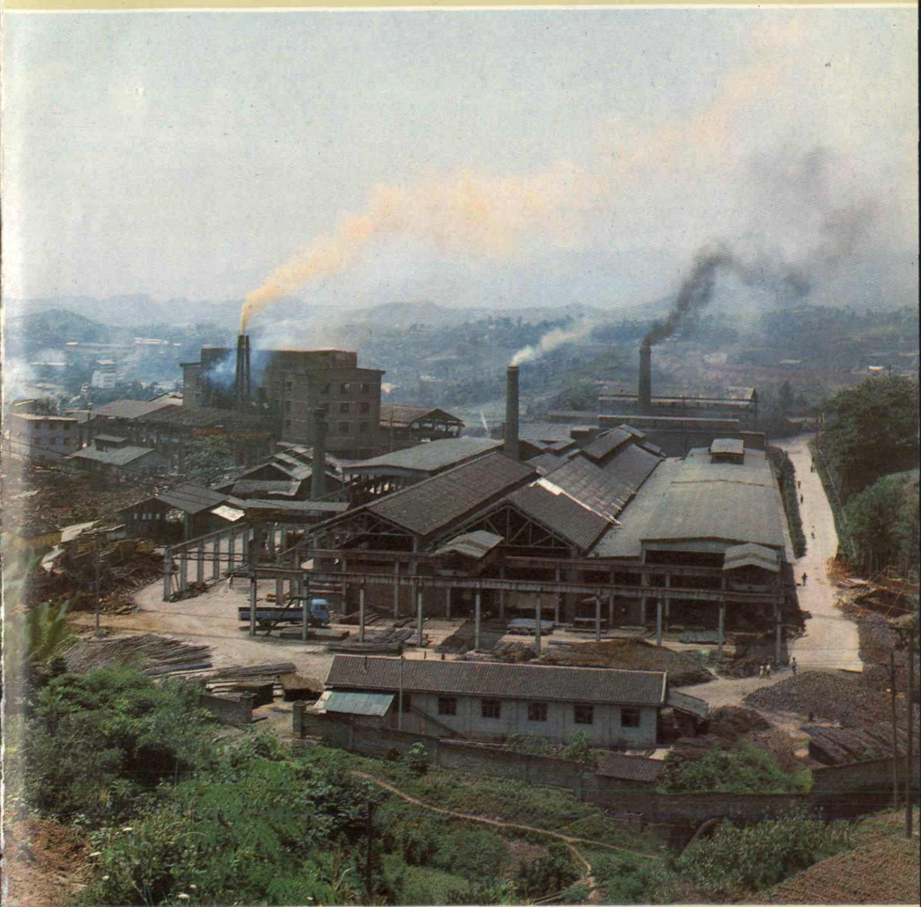
主 厂 房 区 现 貌
