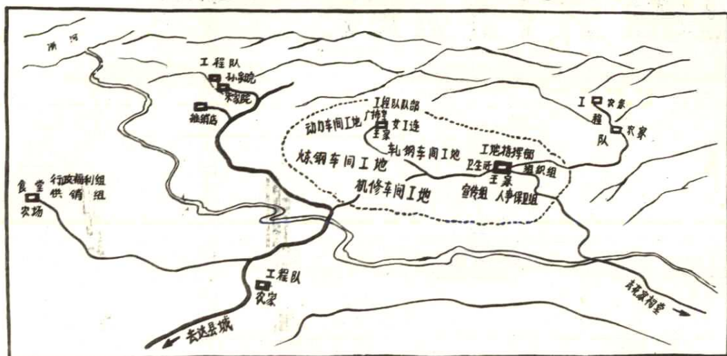
达县红旗钢铁厂王家塆分厂工地示意图
