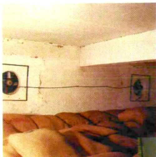
▲ 粮仓轴流式排风储粮
