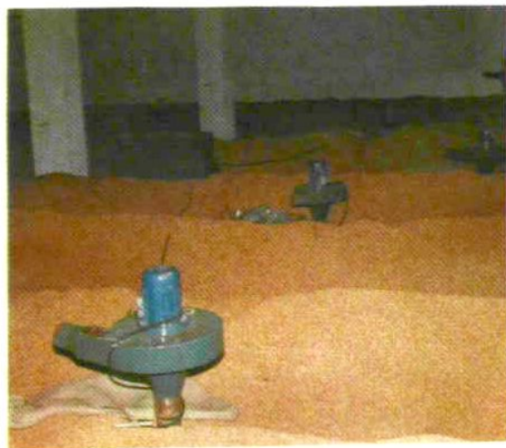
▲ 单管机械通风降温
