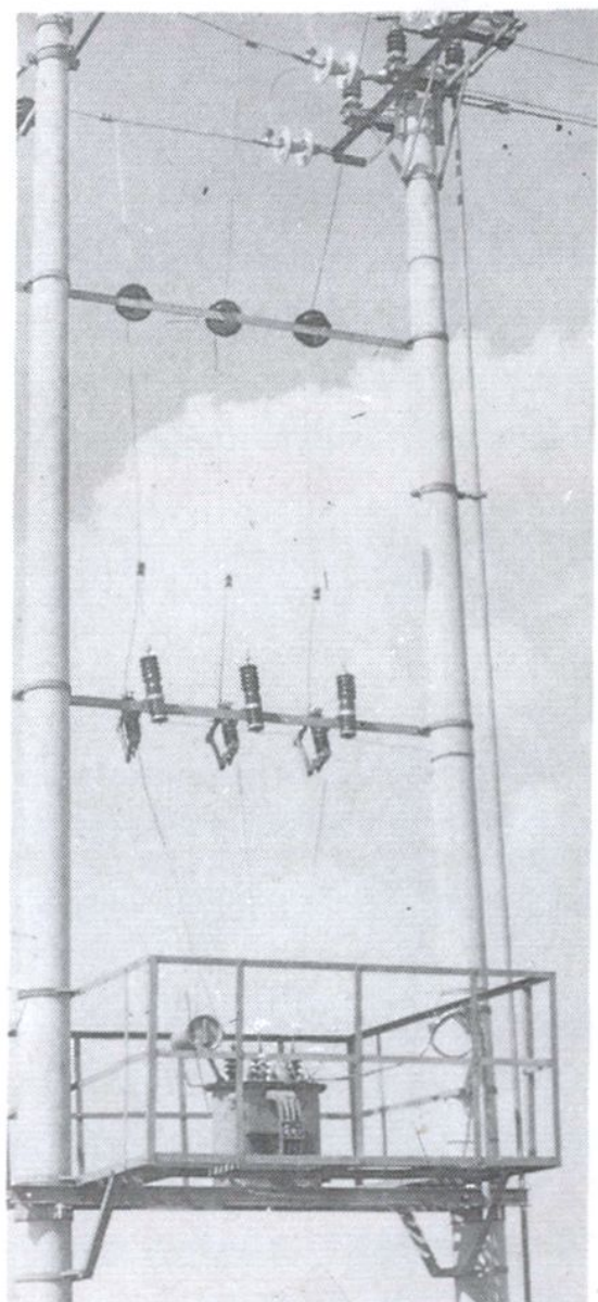
自动闭塞电力杆上设备
