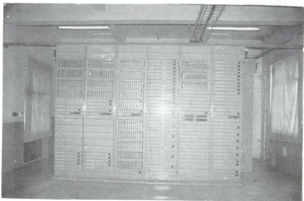
通信自动总机
