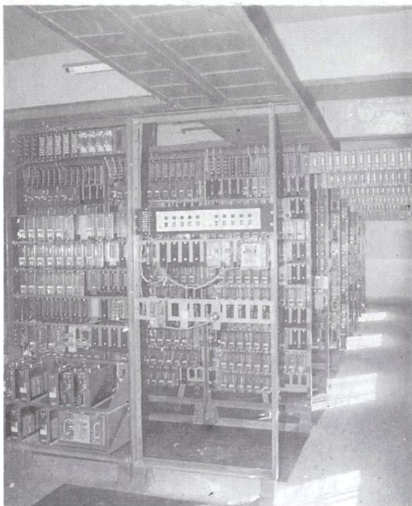
电气集中组合架
