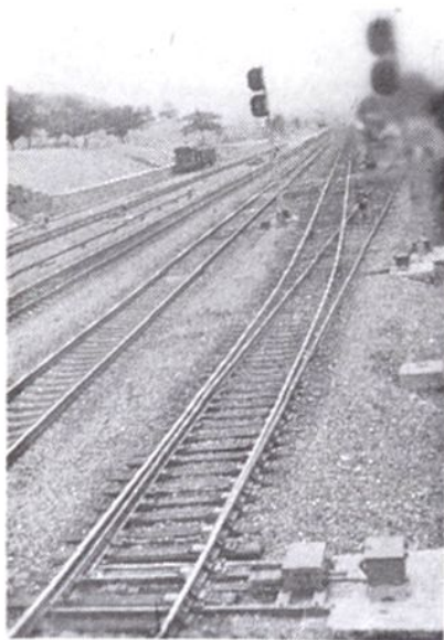
电气集中站内信号设备
