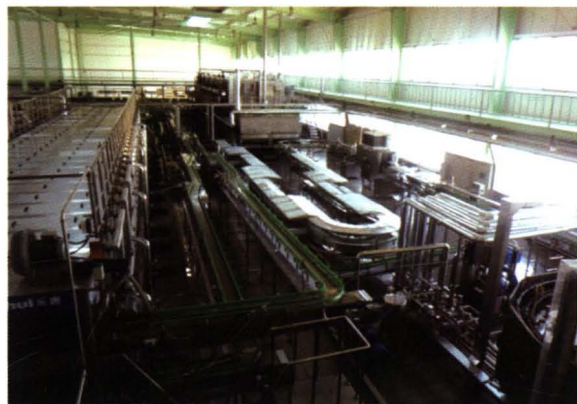
银瀑啤酒罐装生产线
