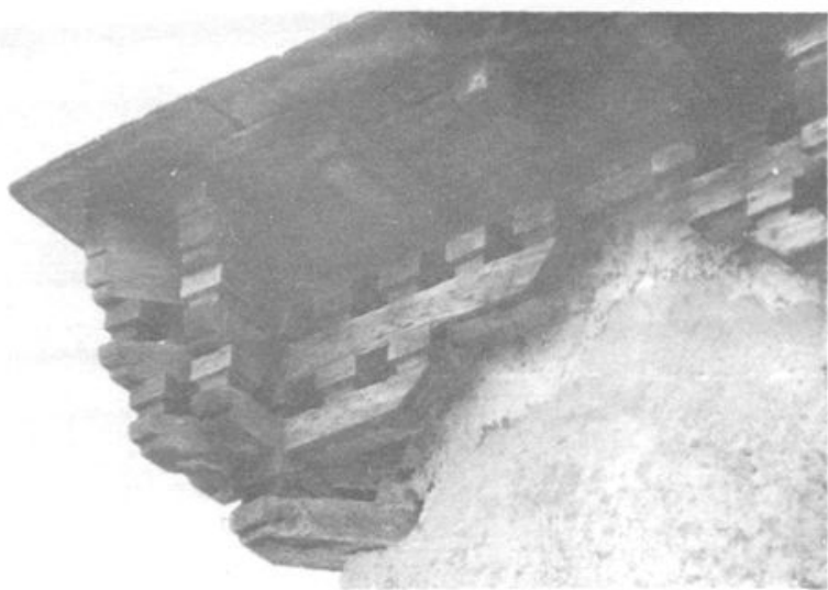
图版二十八 丢热寺大殿檐角斗拱
