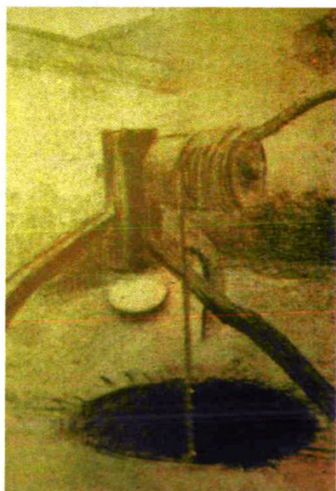
旧时的小煤窑提升辘轳
