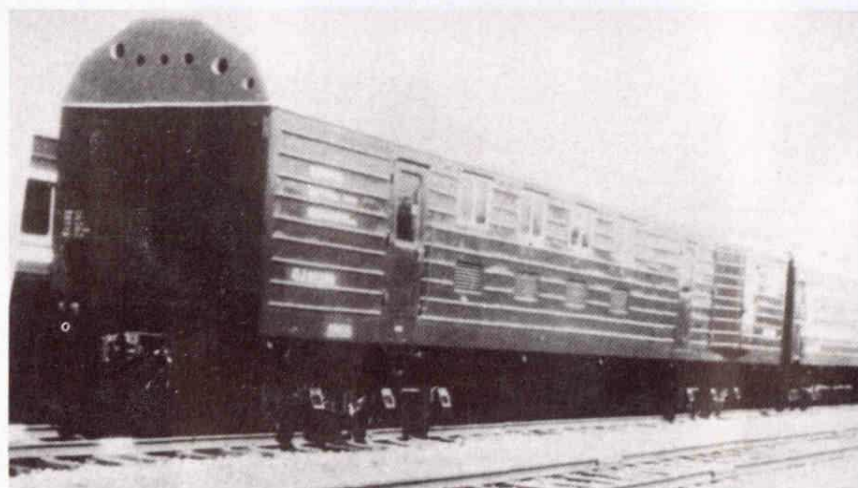
工厂设计生产的 6000KW 蒸汽电站列车——配电车
