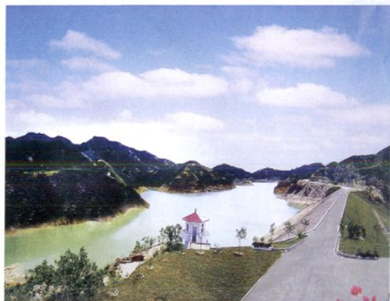
◎ 1998年6月，洪灾后加固的茶山坑水库主坝。
