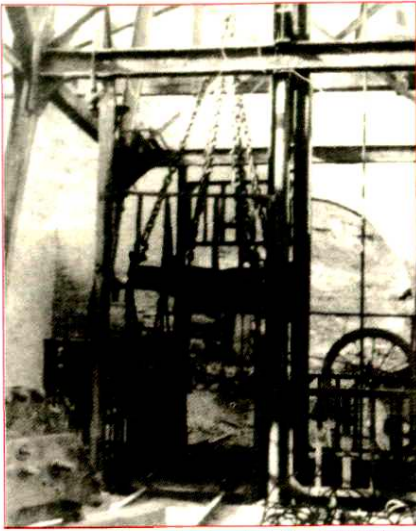
保晋公司第二矿厂，东竖井安设的以蒸汽为动力的提升罐笼
