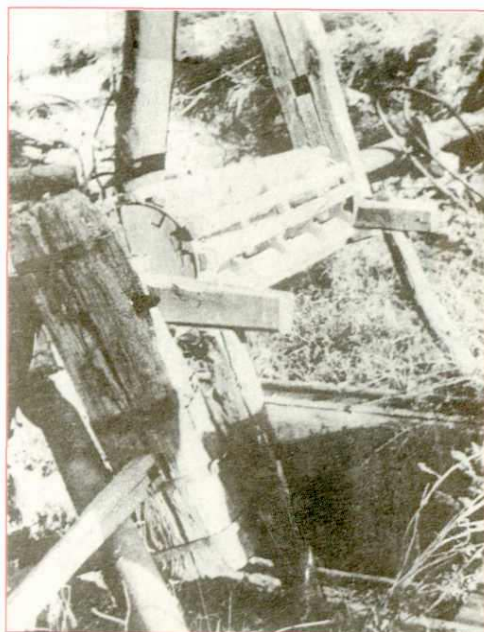
清末民初，晋中一带小煤窑（竖井）提升设施——辘轳（人绞）
