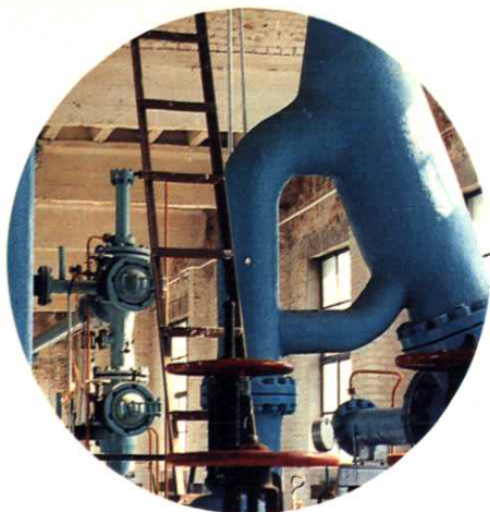
曙光标定站流量计标定装置
