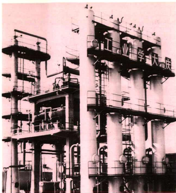
陈家桥脱水站天然气脱水装置
