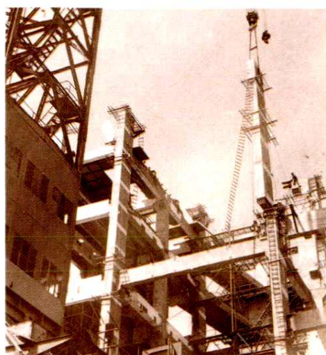
一号机锅炉构架吊装
