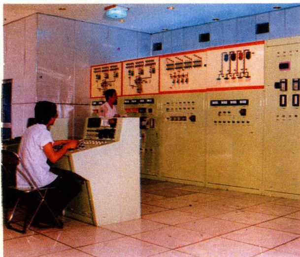
◀密炼机中央控制室◀
