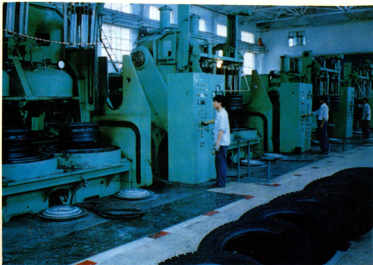
▽双模硫化车间
