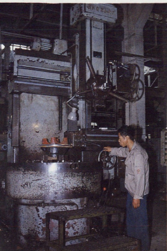
立车
