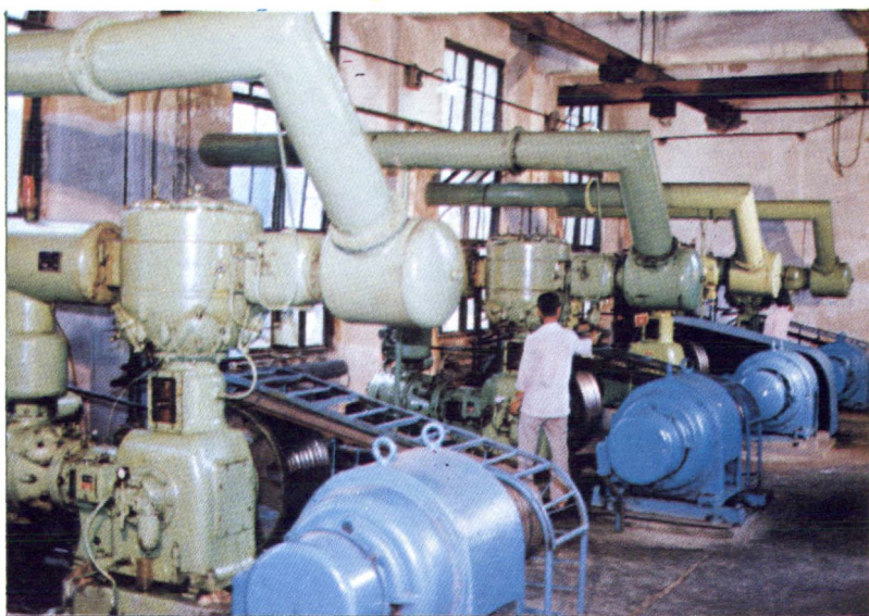
空压站
