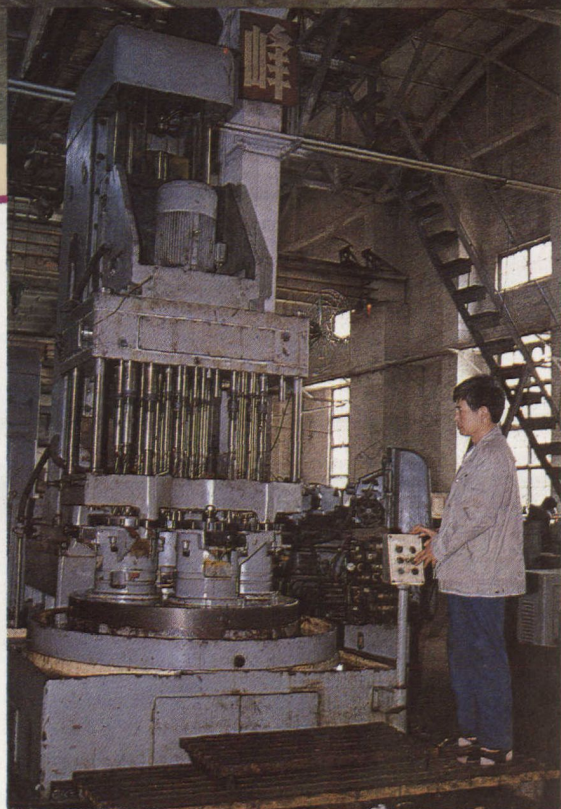
组合机床
