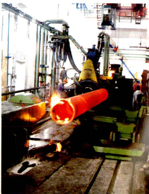
徐钢球墨铸管工程
