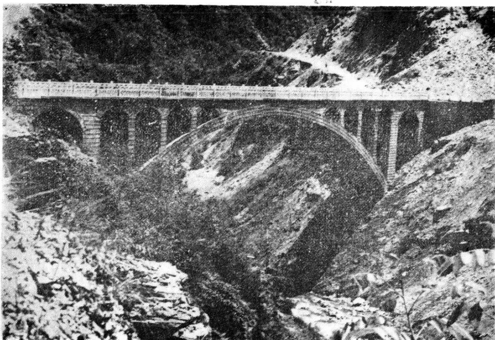
金 凤 大 桥 (图八)
