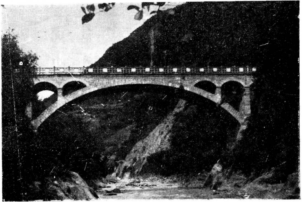
北川县墩上公路石拱桥
