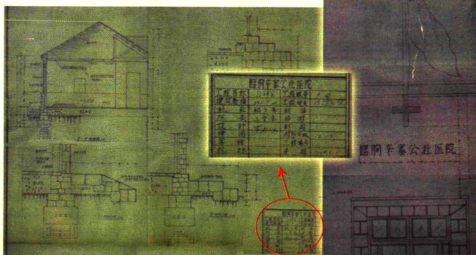
1964年辛寨公社医院门诊工程图纸（局部）
