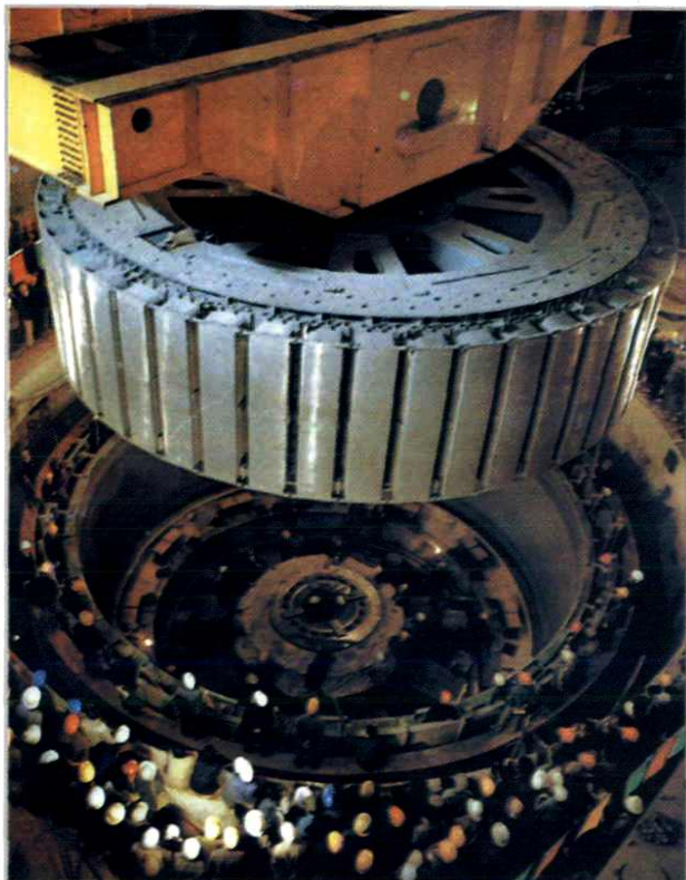
320MW水轮发电机转子吊装
