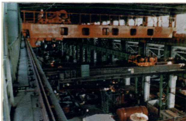
二重厂某车间钢结构厂房之一
