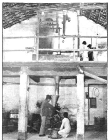
立式95型榨油机
