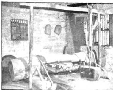
木榨油坊
