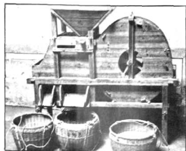
木风车
