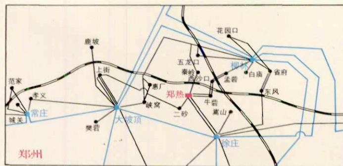
河南省主要城市 110 千伏及以上线路示意图 (1987年)
