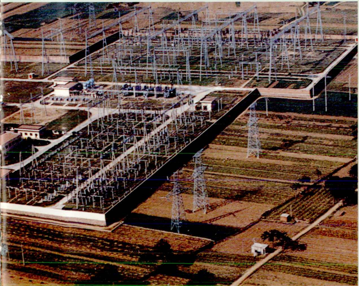
大别山区 110 千伏新县变电站
