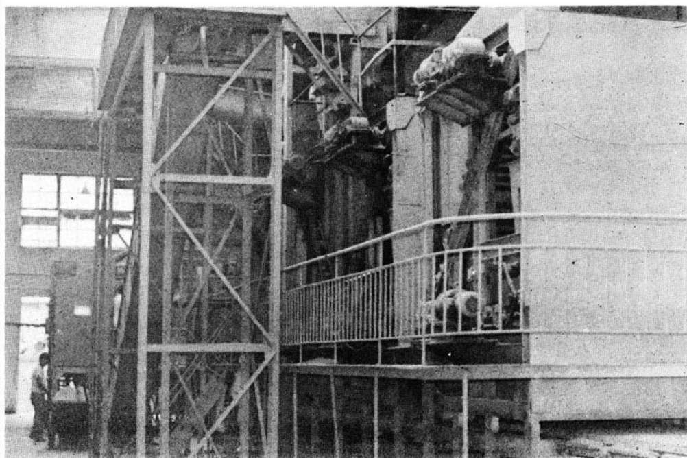
13. 刨花板機器
