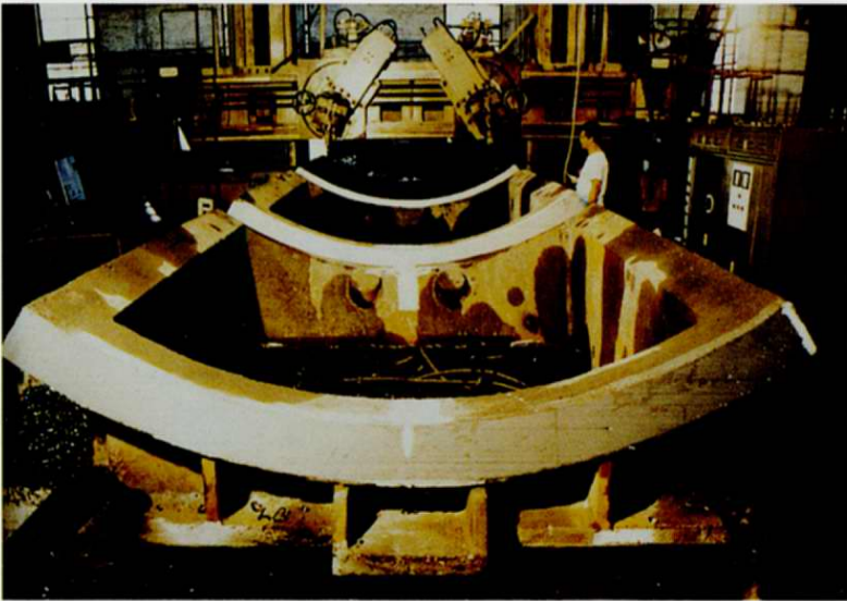
10 米龙门刨床
