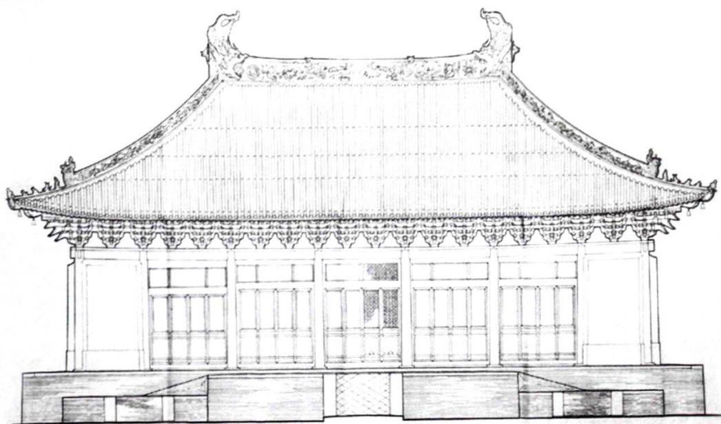
正立面
