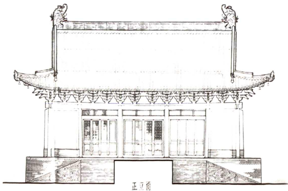
● 龙虎殿正立面图
