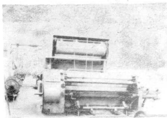
县棉织厂 G142D—180 浆纱机
