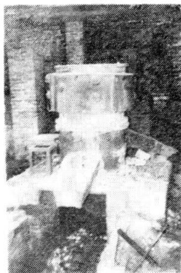
县五金机械厂化铁炉
