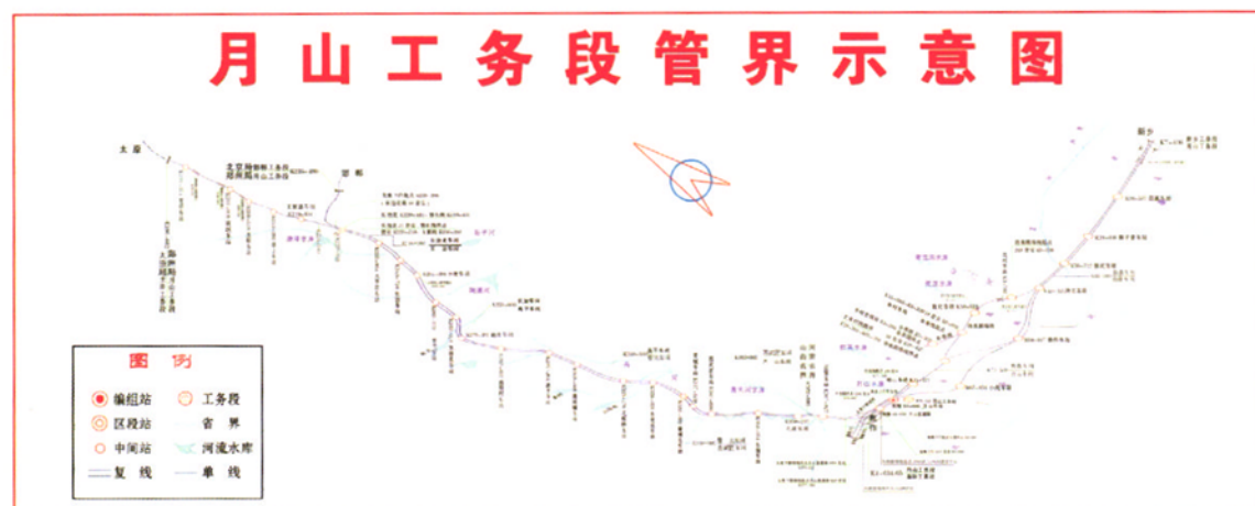
月山工务段管界示意图(2004年11月16日)
