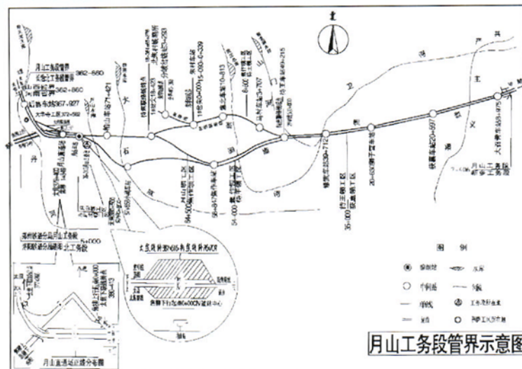
月山工务段管界示意图(2004年11月15日)
