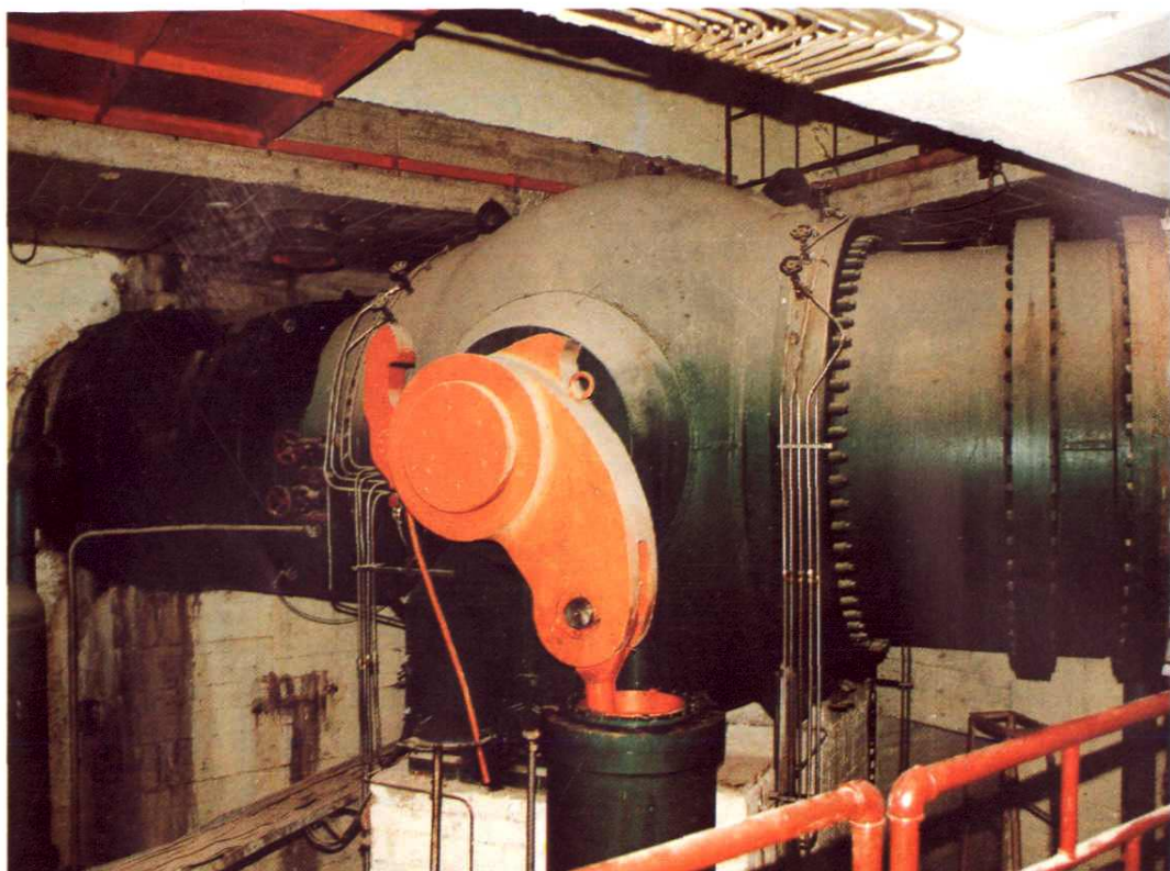
鲁布革电厂球阀
