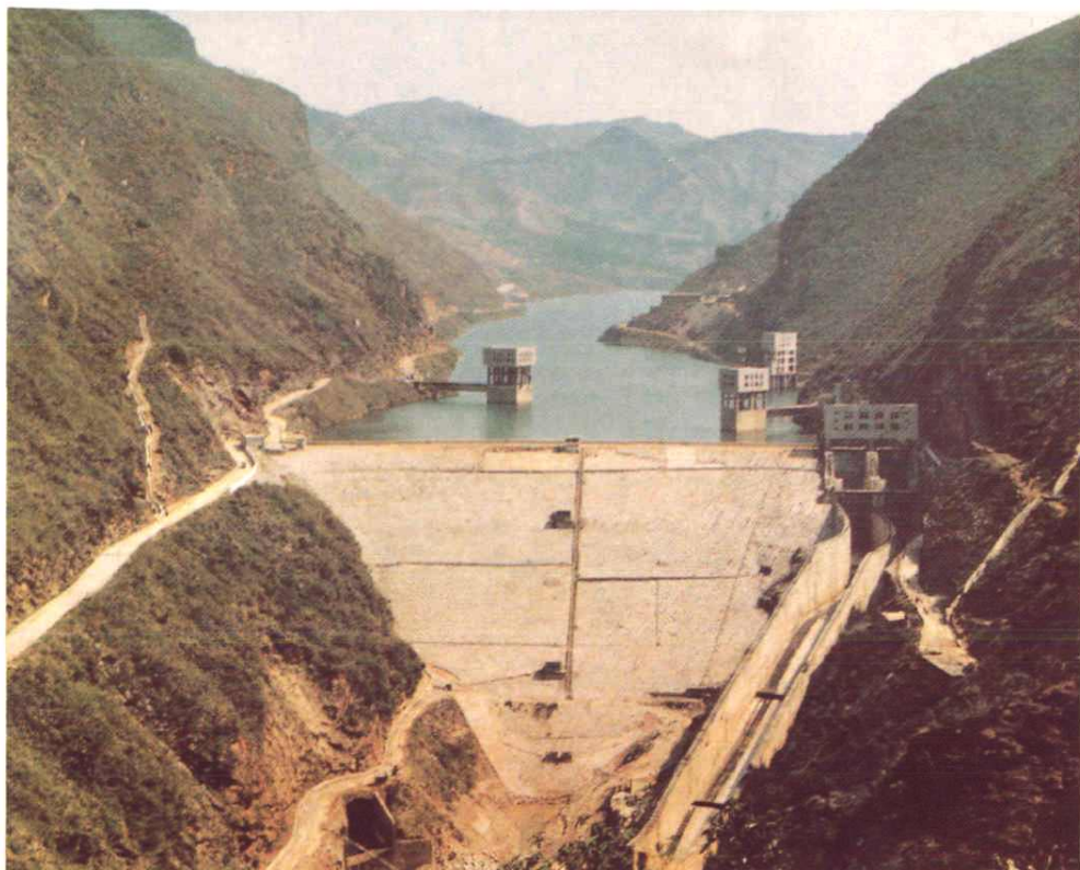
鲁布革电厂大坝
