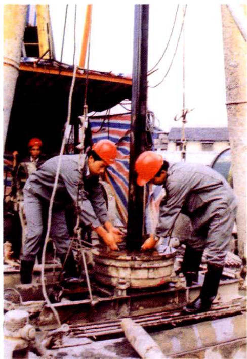
▲ 灌注桩施工场景
