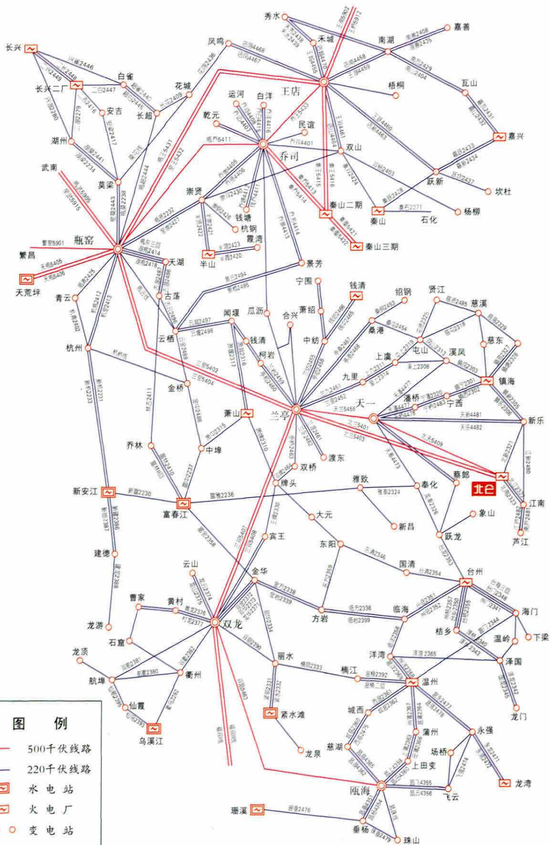
北仑发电厂与浙江电网 220~500 千伏电力系统接线示意图 (2003 年)
