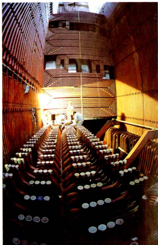
▲ 锅炉水冷壁管安装施工现场
