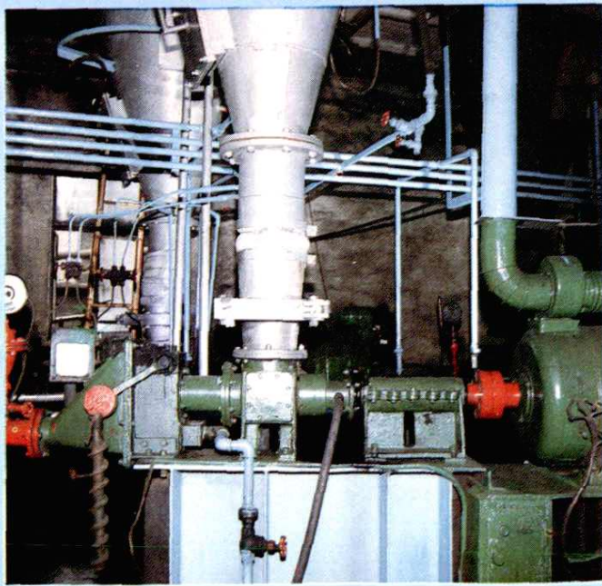
高炉喷煤粉
