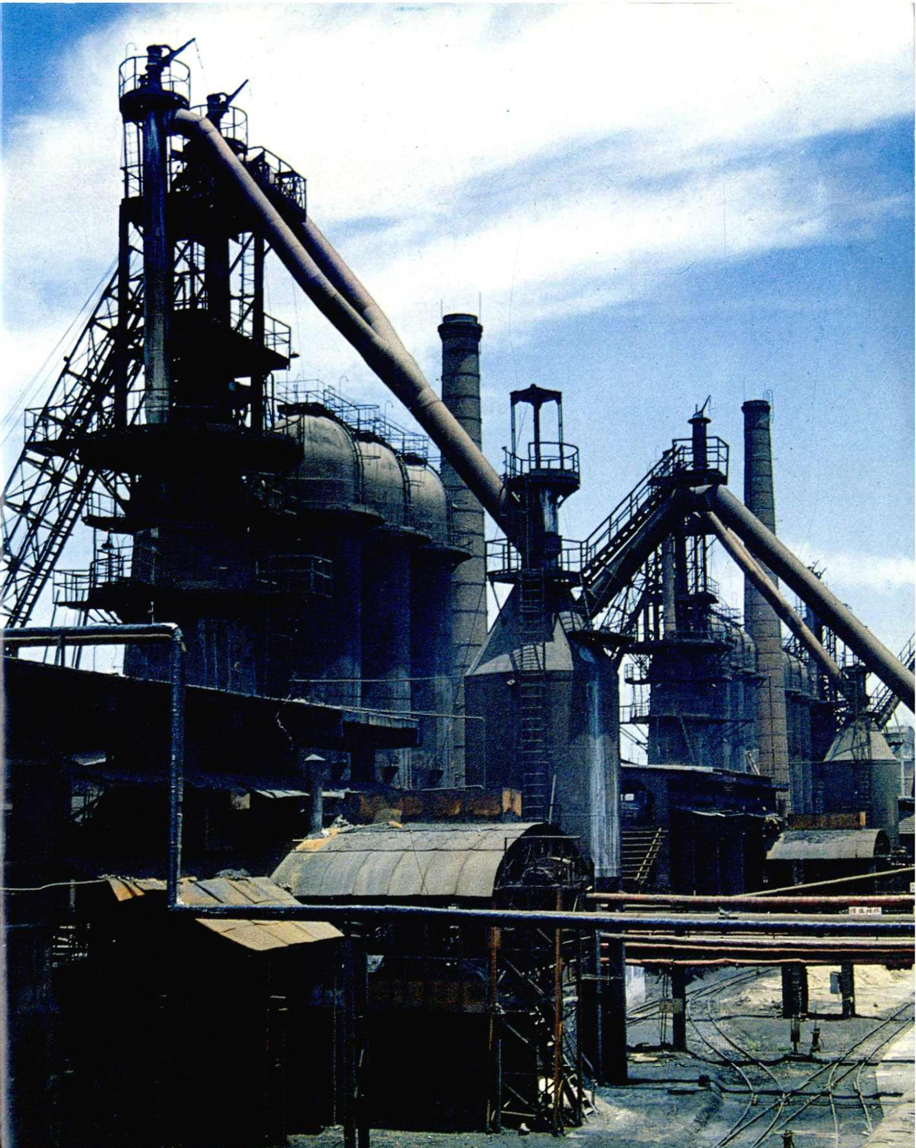
高炉雄姿
