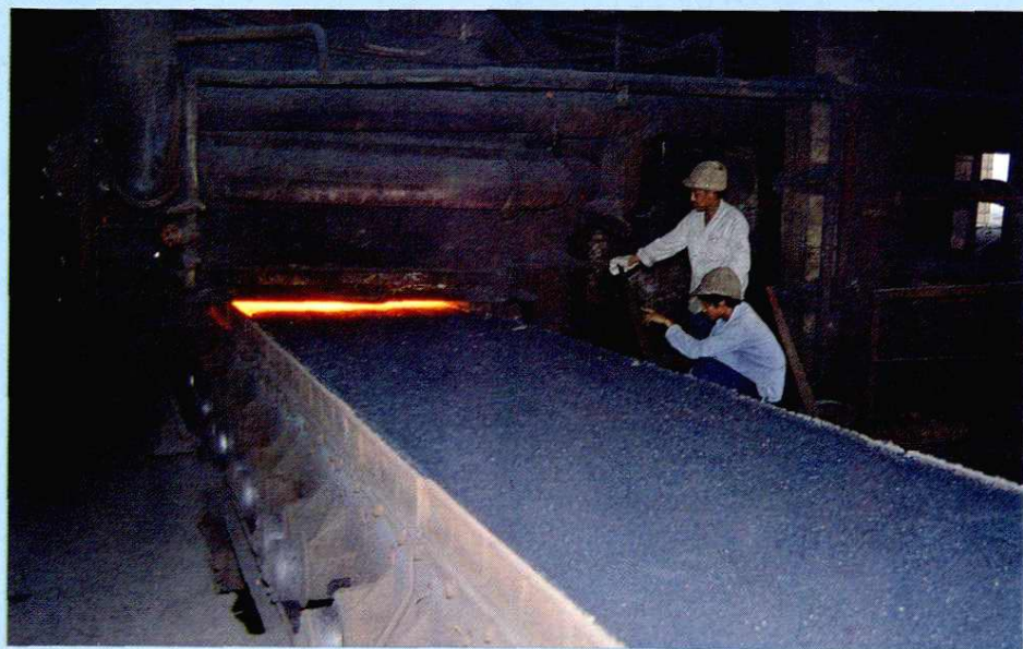
十八平方米烧结机
