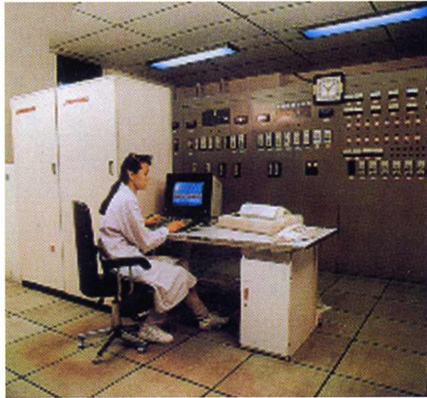
蒸馏主控室
