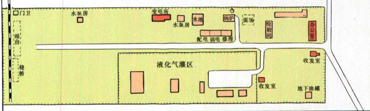
哈尔滨轴承厂厂区总平面图
