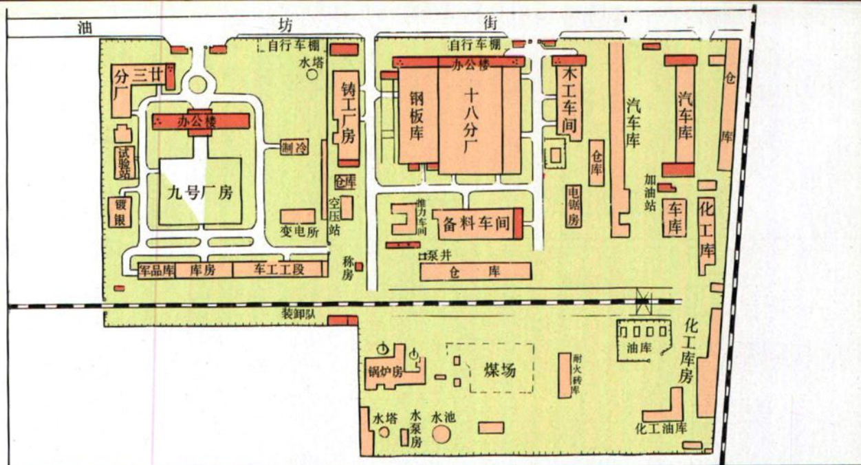
液化气公司平面图 (位于新香坊火车站西南侧)
