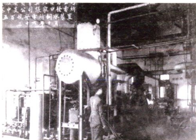
南菜园发电厂饲水车间
