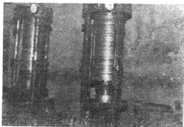
解放前使用的人力土榨螺旋机。
