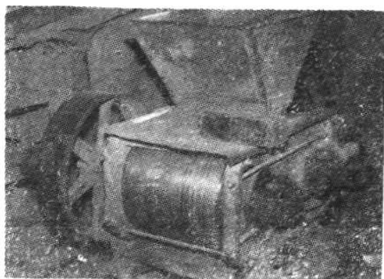
土法榨油使用的花生剥壳机。
