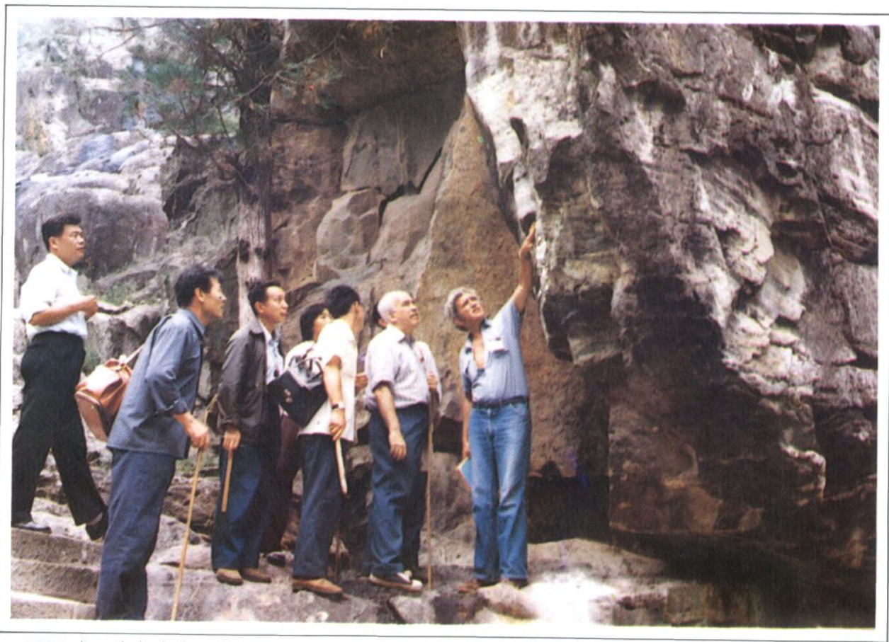
1983 年，我省地质工作者与苏、英等国专家考察泰山经石峪交代混合岩。
