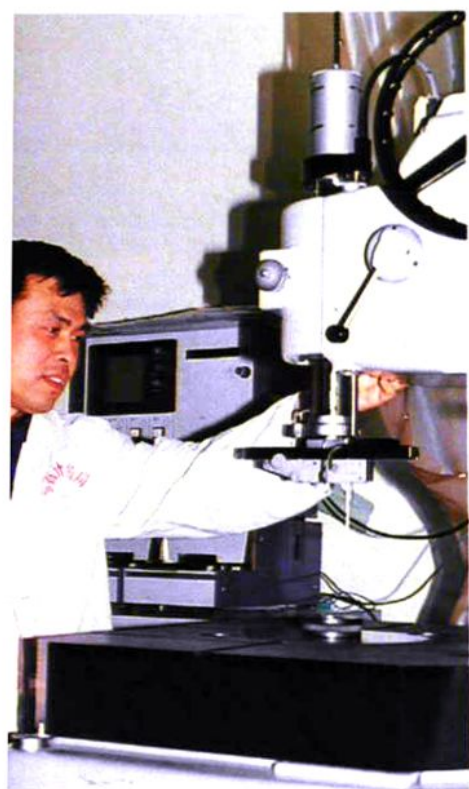
测量圆度
