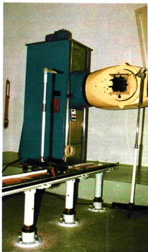
^{60}\text{Co} \gamma 射线标准测量装置
