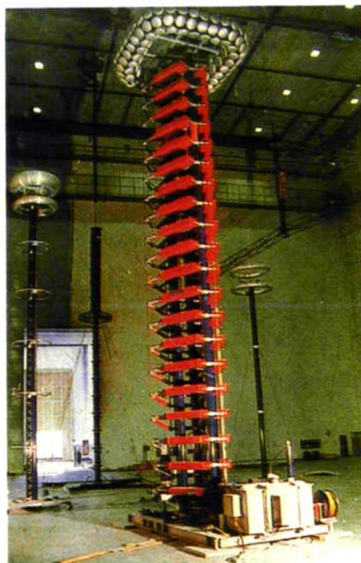
国家高电压计量站的 1000 千伏冲击电压发生器及测量系统
