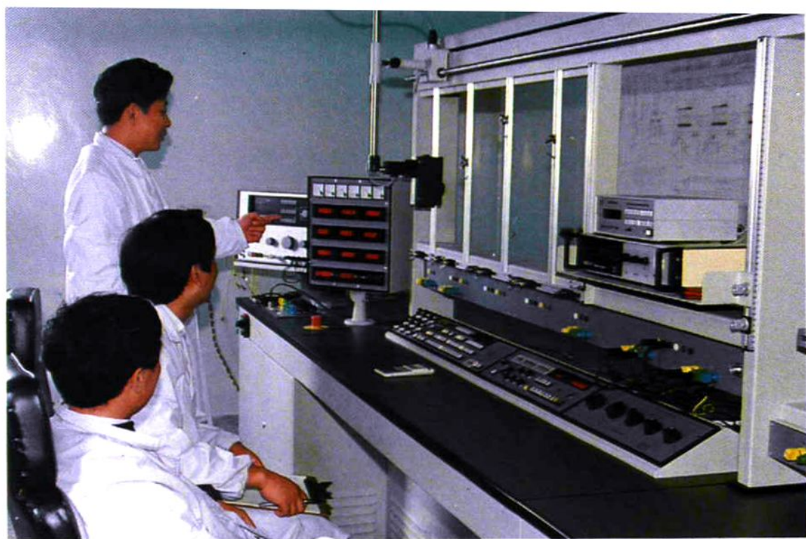
ED7516 型三相电能表校验台
