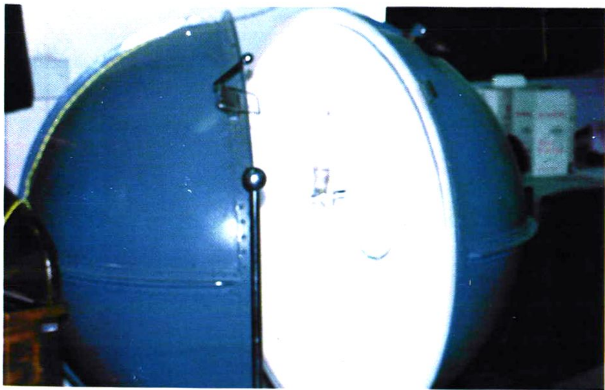
积 分 球
