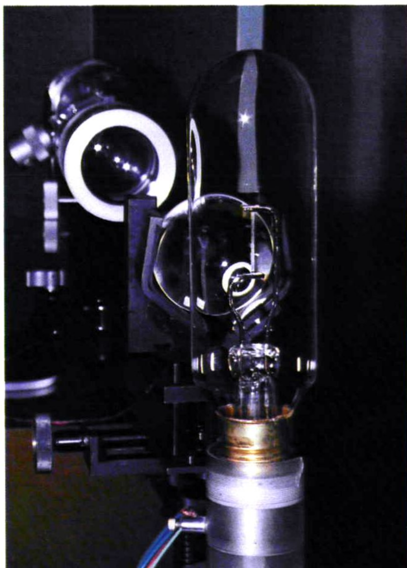
标准温度灯检定装置
