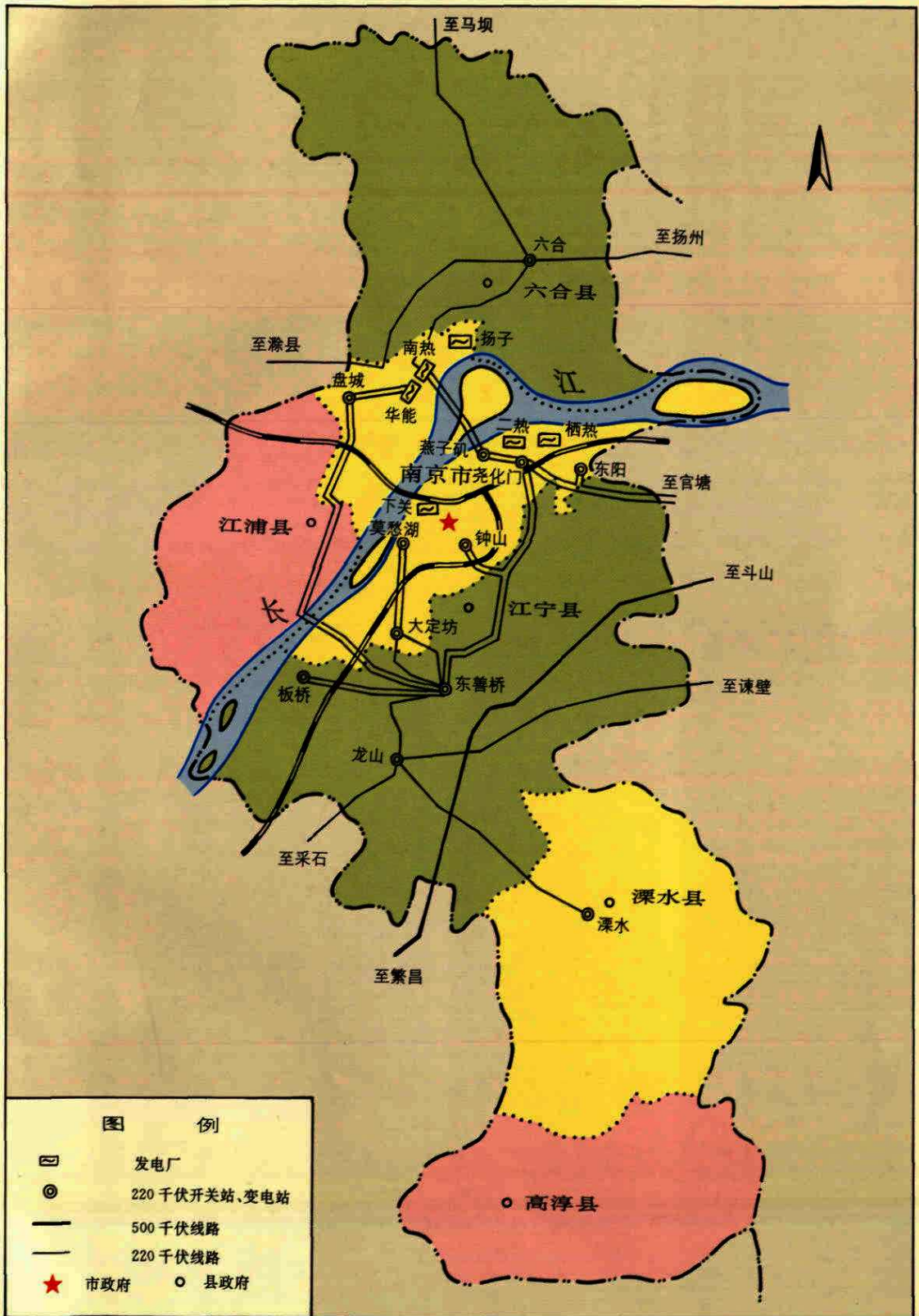
南京电网地理接线示意图 (1995年)
