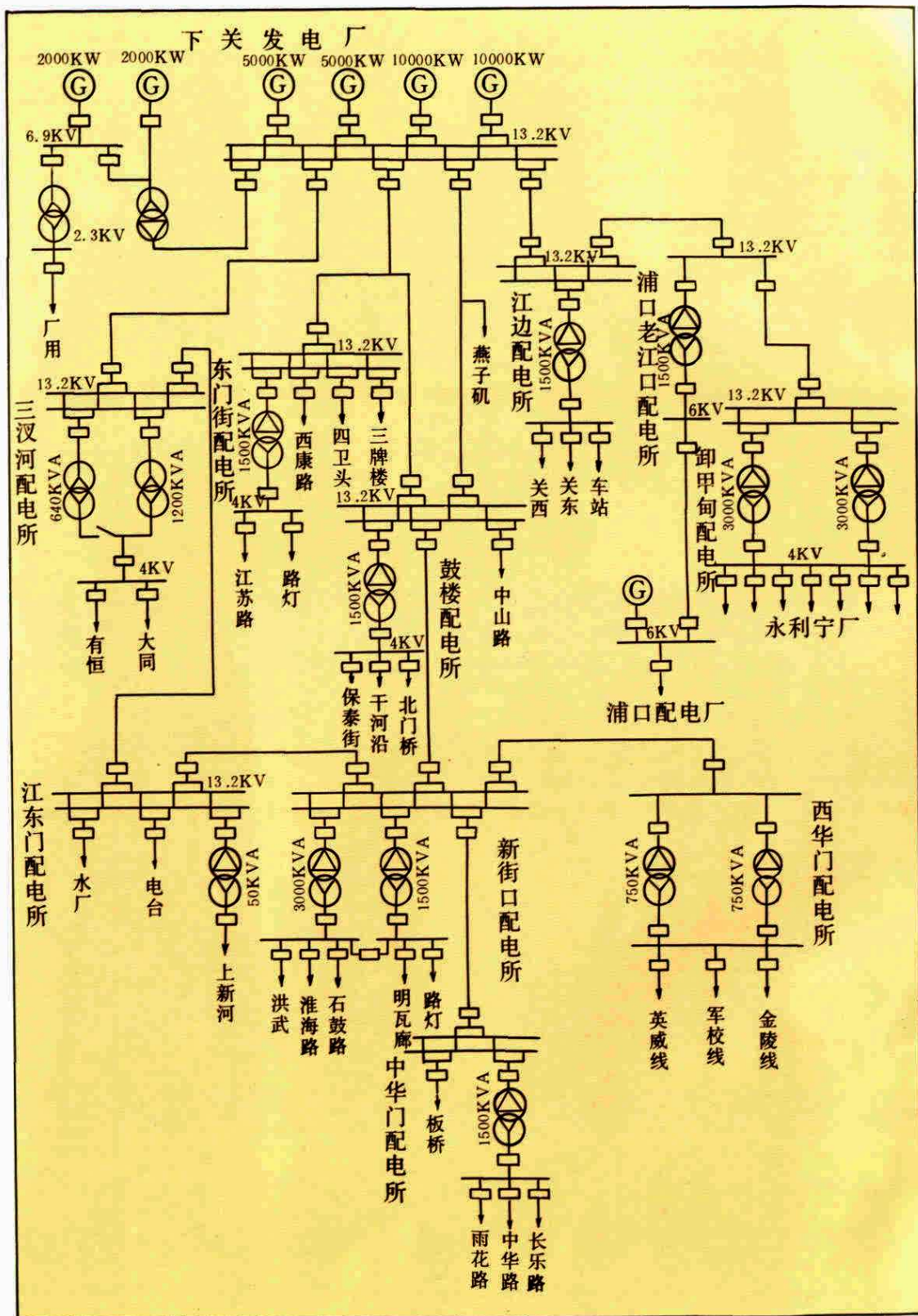
南京送配电线路系统图 (1949年4月)
