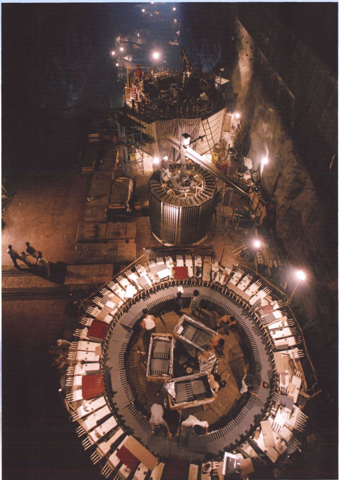
1994 年，天荒坪抽水蓄能电站主厂房水轮发电机组安装现场
