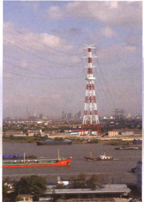
2001年12月开工建设的 上海500千伏输电线路吴淞口 黄浦江大跨越塔
