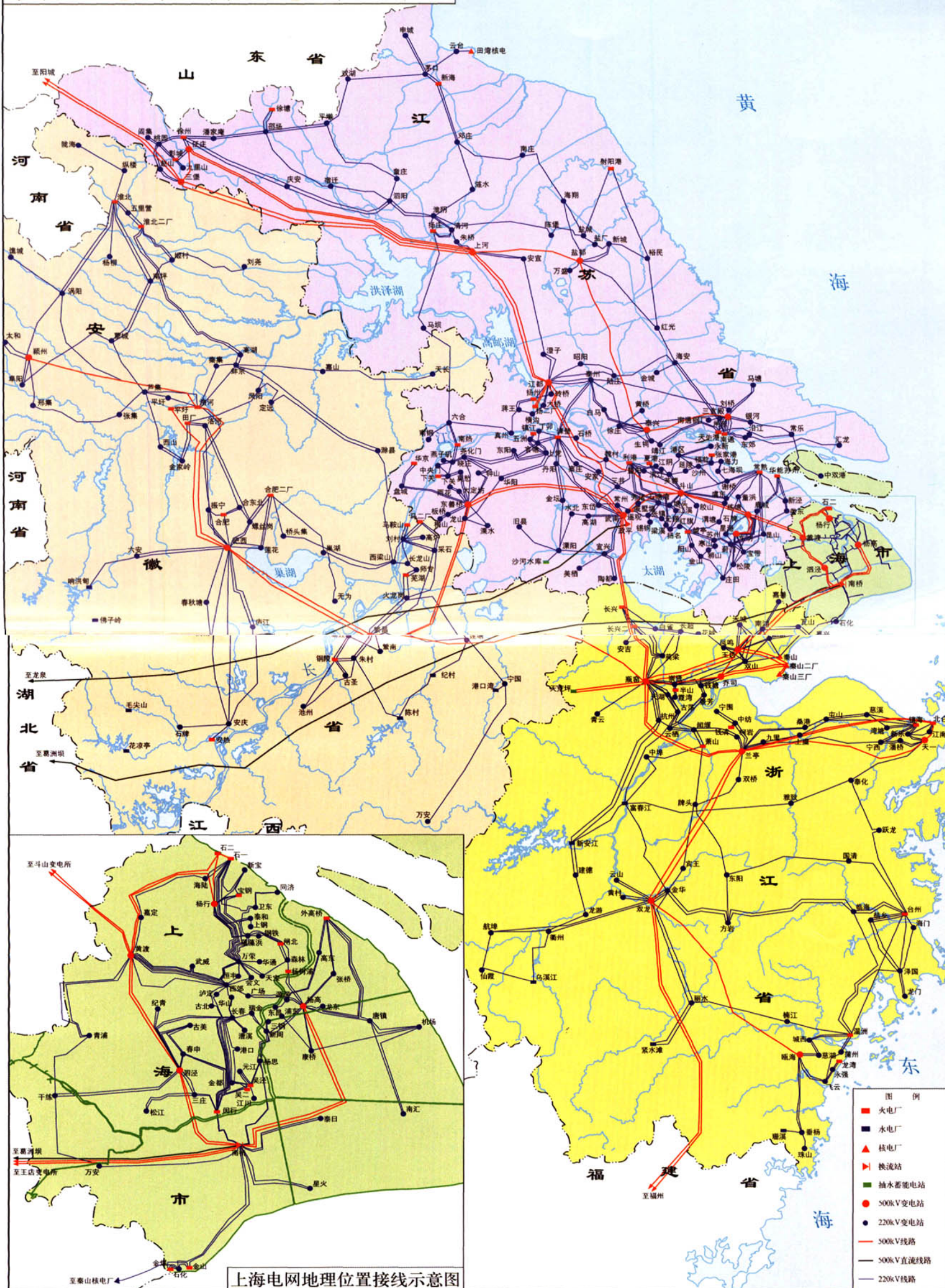
华东电网地理位置接线示意图(2002年底)
