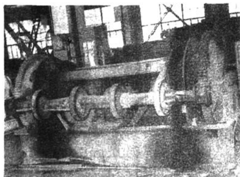
自制1.5吨矿车成型机(1979年)
