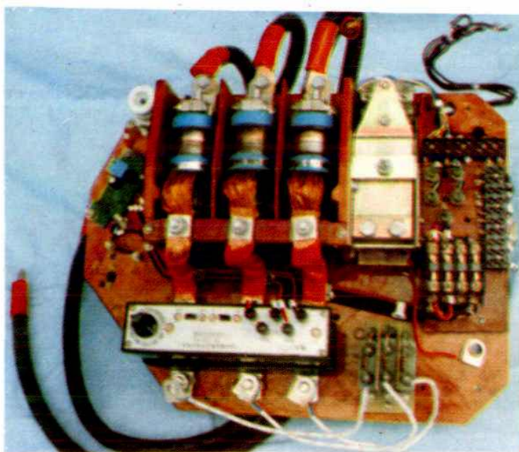
电器仪表
