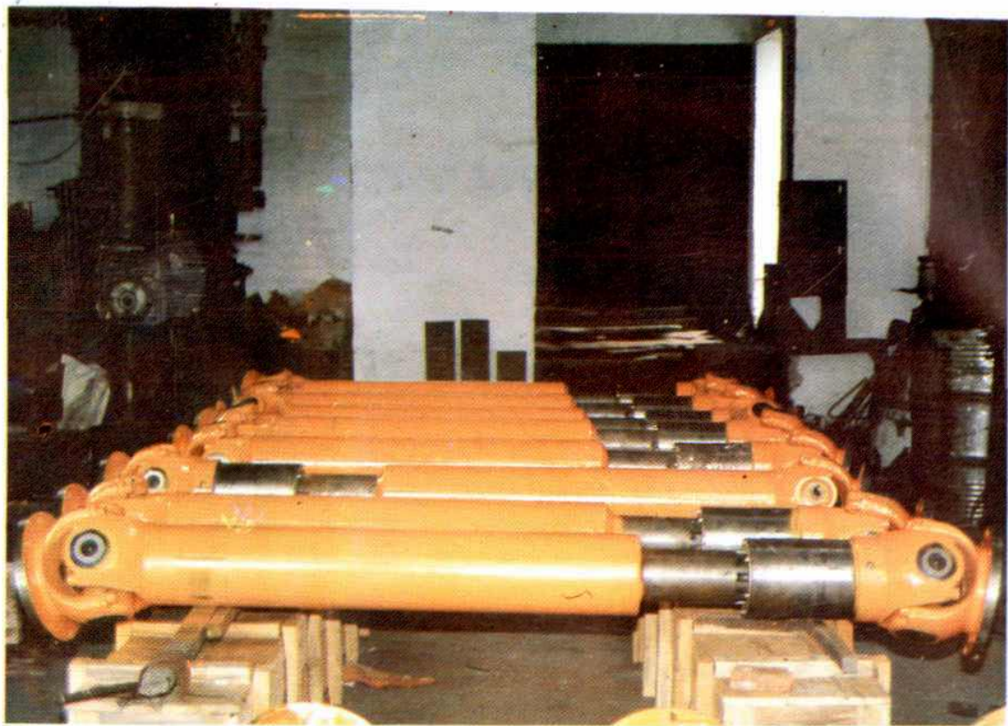
万向联轴器
