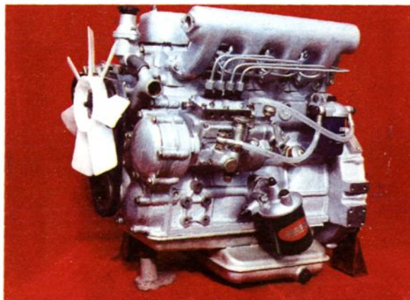
▽江发总厂研制的F485型柴油机
