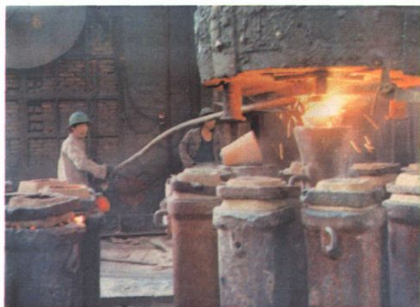
沈阳钢铁总厂炼钢车间在注锭
