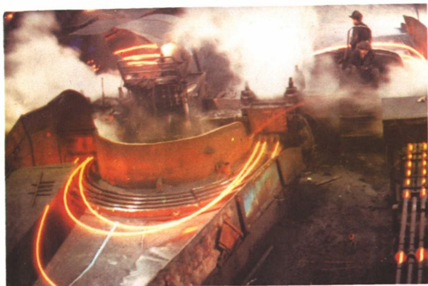
沈阳线材厂线材生产
