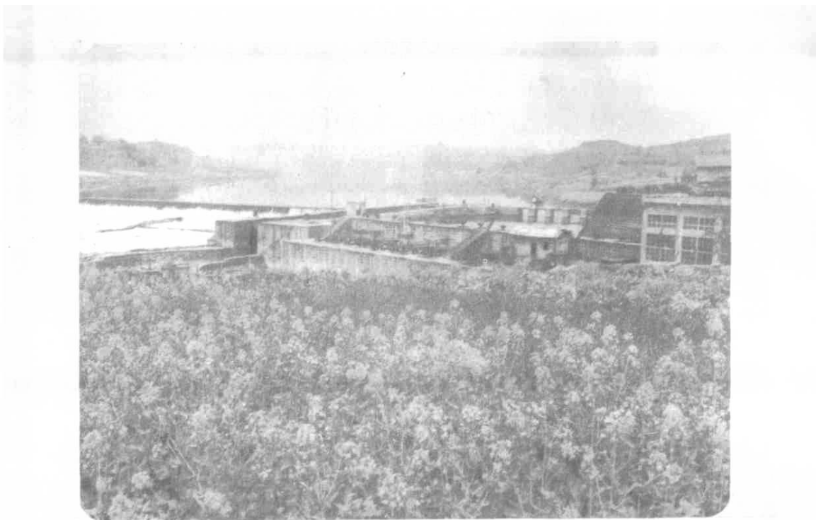
隆昌县兴建的石盘滩水轮泵站，是沱江干流上第一座拦河筑坝提灌工程（简称沱灌工程）。年提水量一亿立方米。图为水轮泵站全貌。
