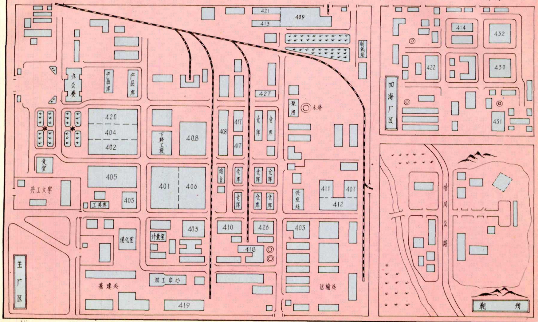
国营哈尔滨第一机器制造厂示意图
