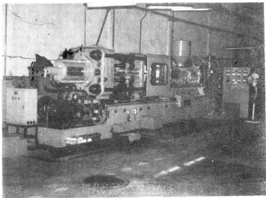
一千克塑料注射机
