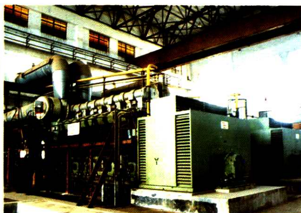
1994年吴川光华电厂引进2×1.12万千瓦柴油发电机组
