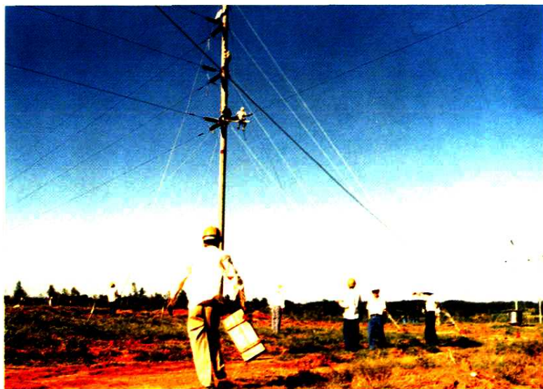
雷州市农网改造现场
