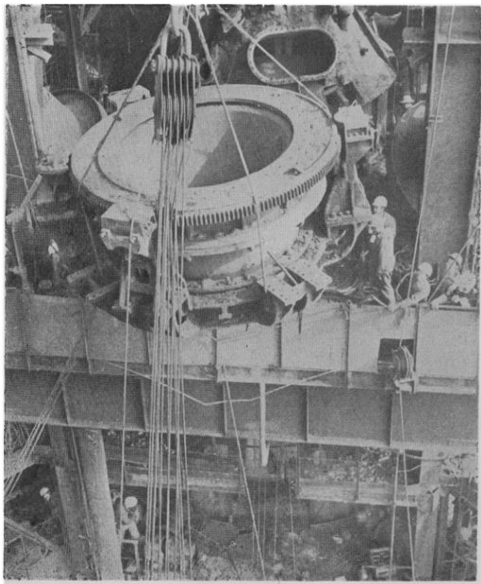
吊 装 高 炉 布 料 器
