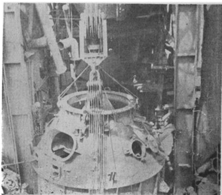
吊装高炉大小钟及保护罩
