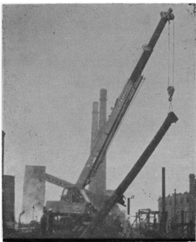
焦炉大修：16吨液压吊上焦炉炉顶作业
