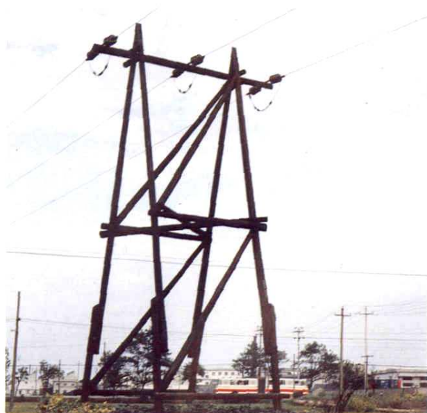
35 千伏杭州—海宁线路木塔
