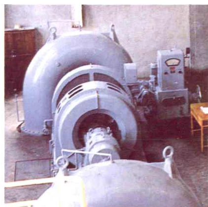
桐庐肖岭二级水电站
