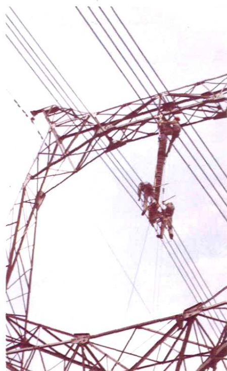
500 千伏线路整串绝缘子更换
