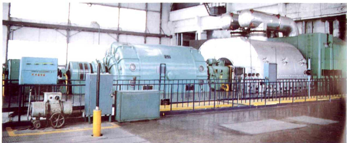
半山发电厂 12.5 万千瓦汽轮发电机组
