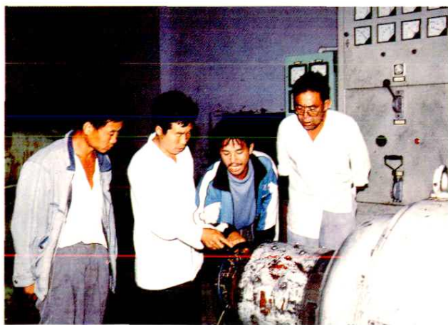
立新村电站320+320+160千瓦电机室
