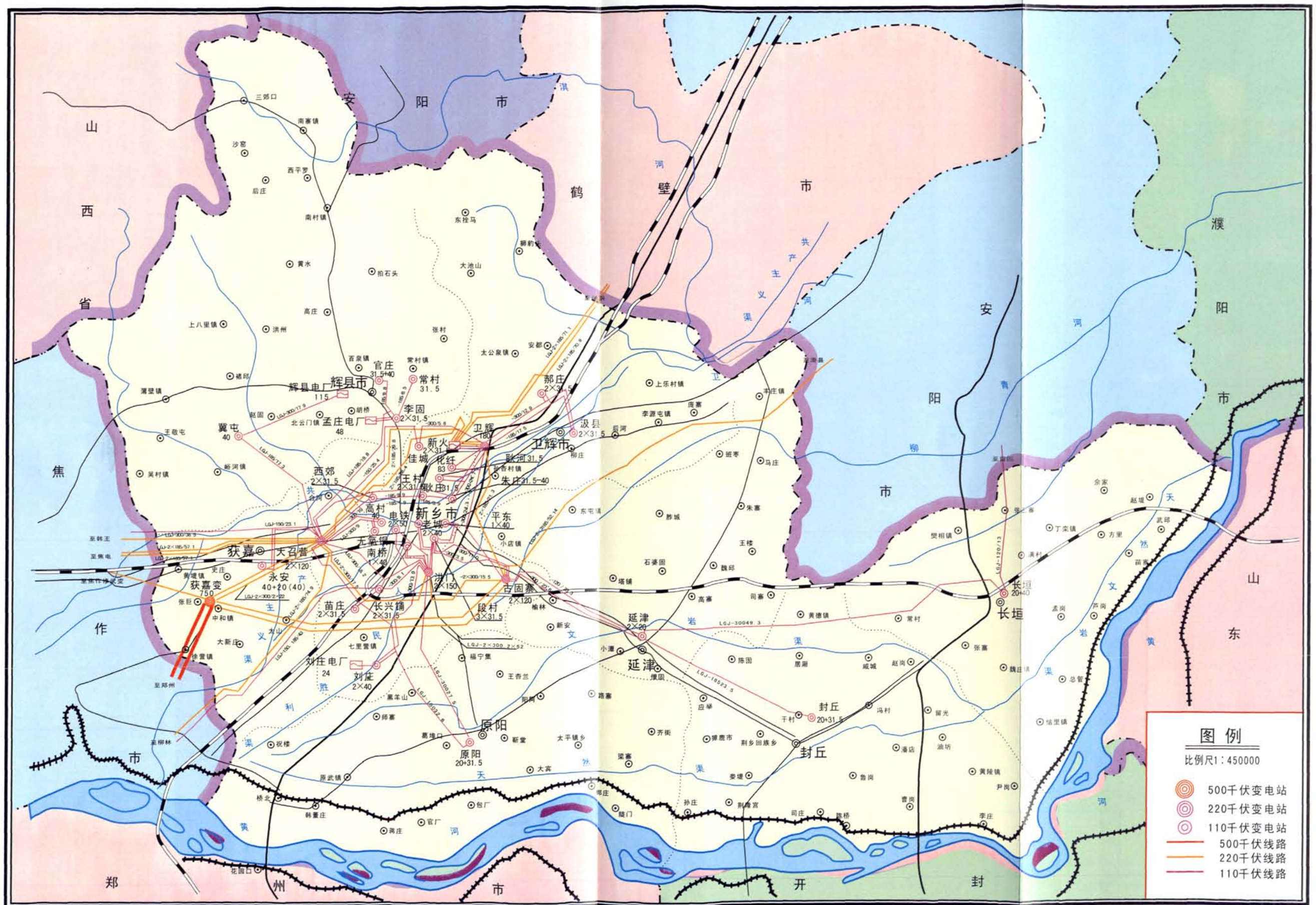
2001年新乡供电区110千伏以上电网地理接线示意图
