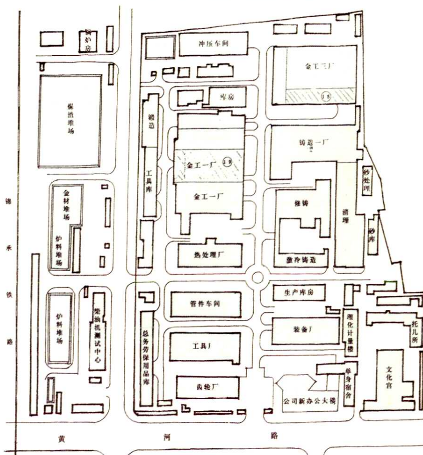
南厂区平面示意图 比例尺: 1: 2900
