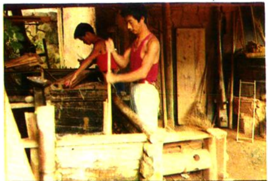
纸农在纸槽生产土纸
